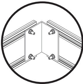
Montage eine Fußleiste
