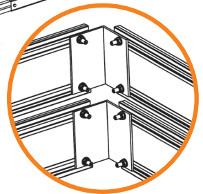
Montage doppelte Fußleiste
